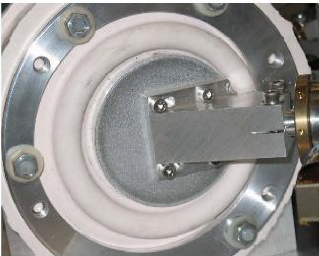
Fig(40-a): Diaphragm pistons
