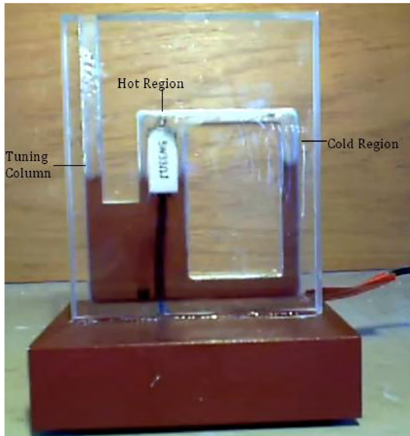
Fig(35): An actual Fluidyne engine.
